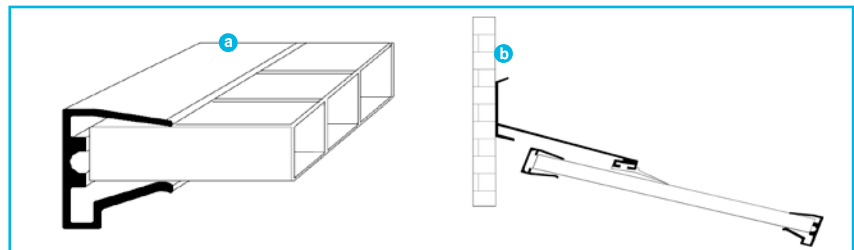
Zu 3.: Alu-Tropfkantenprofil mit Platte sowie Querschnitt WA + T16 + U16
